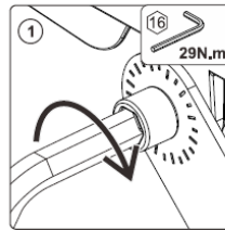
בורג קיבוע מומלץ: M10
