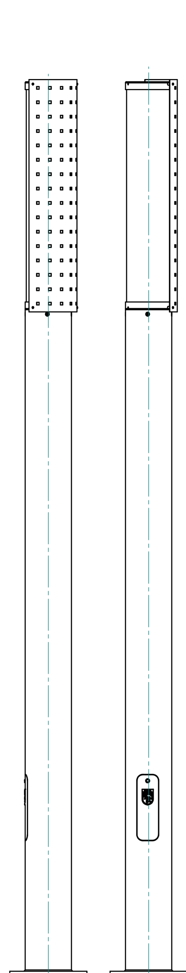
Korintosz Smart Maxi Opál+díszítőlemez (Korintosz_Smart_Maxi_Opál_díszítőlemez_3+1m.stp) - 3m oszlop; 1m világítóegység - Henger alakú, ütésálló Opál műanyag bura - Színhőmérséklet: 3000 v. 4000K - Opciók: LED szalag (RGB) - Díszítőlemez akár egyedi design alapján - Választható RAL szín
