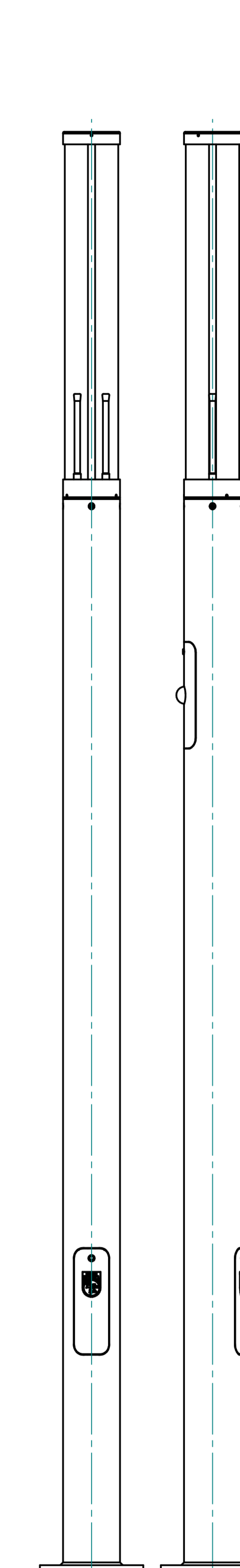
Korintosz Smart Midi+WiFi+Kamera (Korintosz_Smart_Midi_WiFi+Kamera_3+1m.stp) - 3m oszlop; 1m világítóegység - Henger alakú, ütésálló Vízizsuga műanyag bura - Színhőmérséklet: 3000 v. 4000K - Választható RAL szín
