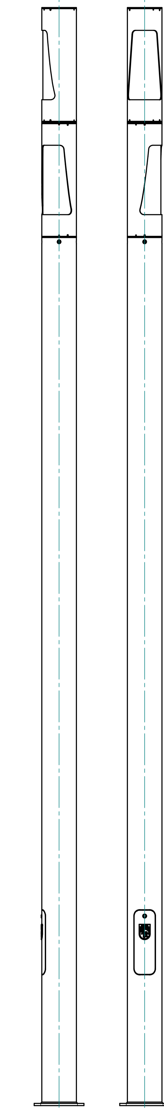
Mobile (Mobile_4+2x0,5m.stp) - 4m oszlop; 2x0,5m irányított világítóegység - Henger alakú, ütésálló Vízizsuga műanyag bura - Színhőmérséklet: 3000 v. 4000K - Választható RAL szín
