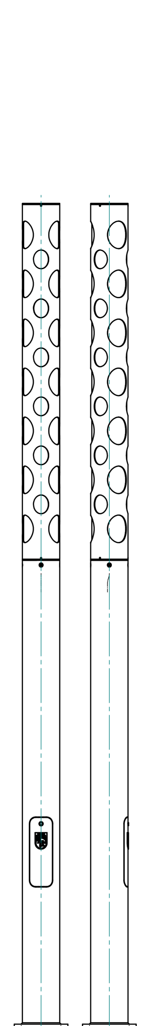
Korintosz Smart Midi lona (Korintosz_Smart_Midi_lona_Teljes_összeállítás_2+1,5m.stp) - 2m oszlop; 1,5m világítóegység - Henger alakú, ütésálló Opál műanyag bura - Színhőmérséklet: 3000 v. 4000K - PCB - Választható RAL szín
